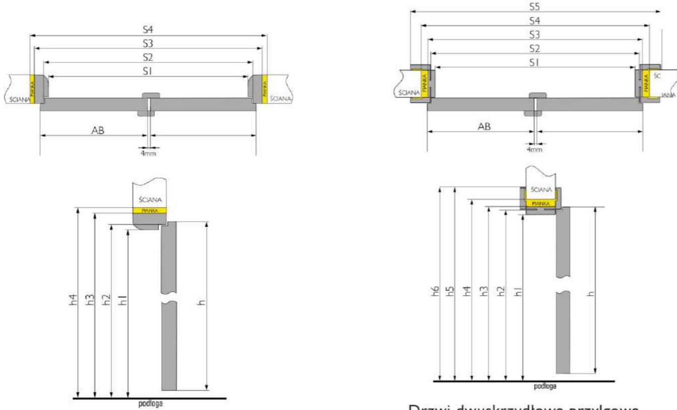
Drzwi dwuskrzydłowe przylgowe z ościeżnicą regulowaną OP/OS
